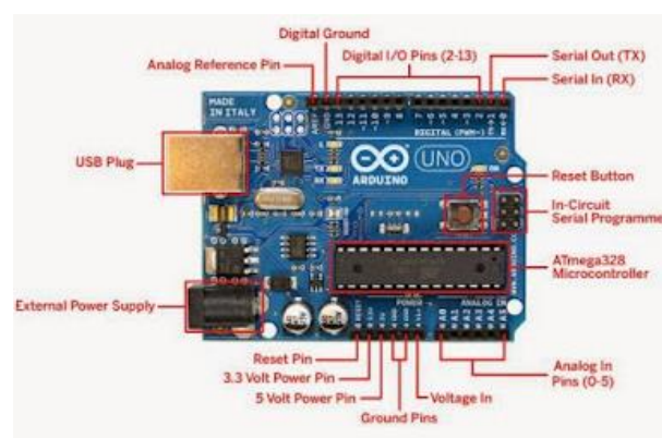
Gambar 1. Arduino Uno [4]
