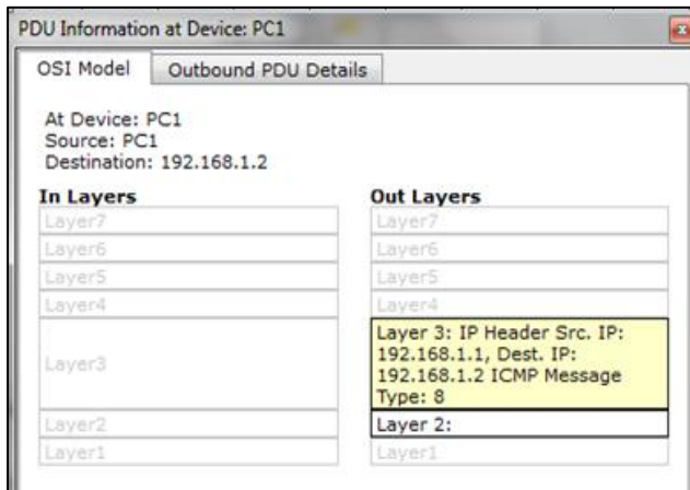
Gambar 4. ICMP Packet dari PC1
