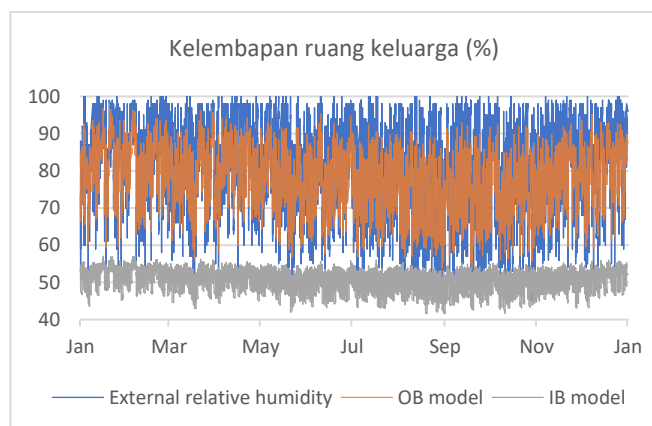
Gambar 13. Perbandingan kelembapan ruang keluarga antara model bangunan studi kasus (OB) dengan bangunan dengan insulasi (IB).
