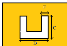
Gambar 3. Bentuk U-Slot pada patch antenna mikrostrip.
