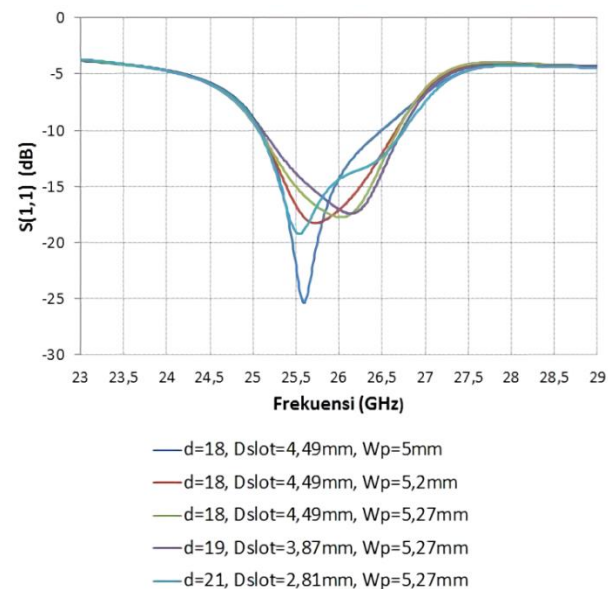
Gambar 7. Optimasi S(1,1) antenna mikrostrip tunggal dengan double U-slot patch .
