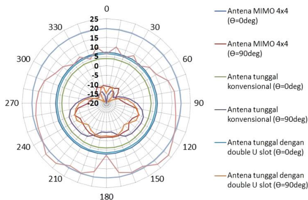
Gambar 20. Hasil pola radiasi azimuth antenna mikrostrip tunggal dan MIMO 4×4.
