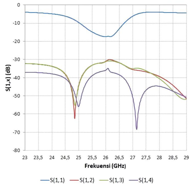
Gambar 12. Hasil S-Parameters antenna mikrostrip MIMO 4 \times 4 dengan double U-slot patch dan DGS elemen ke-1.
