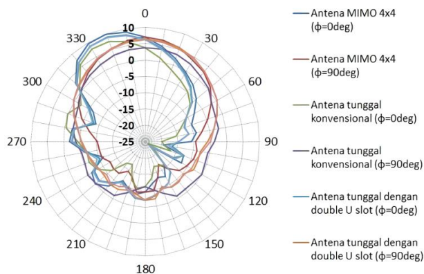
Gambar 19. Hasil pola radiasi elevasi antenna mikrostrip tunggal dan MIMO 4×4.
