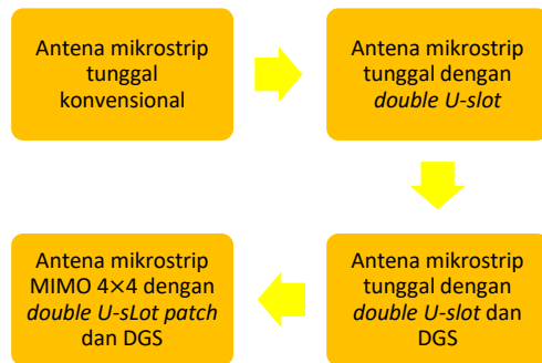
Gambar 5. Diagram alir perancangan antenna mikrostrip MIMO 4×4 dengan double U-Slot patch dan DGS.
