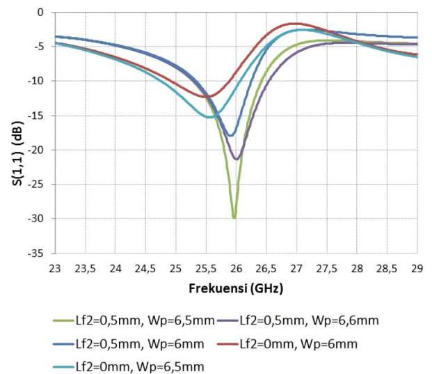
Gambar 6. Optimasi S(1,1) antenna mikrostrip tunggal konvensional.
