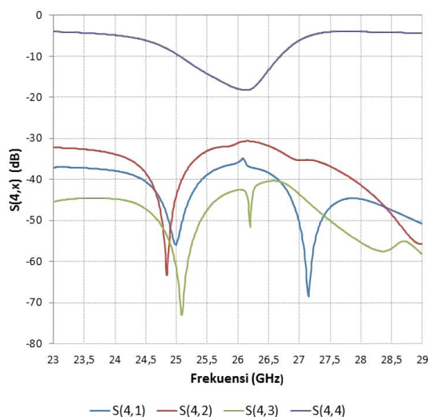
Gambar 15. Hasil S-Parameters antenna mikrostrip MIMO 4×4 dengan double U-slot patch dan DGS elemen ke-4.
