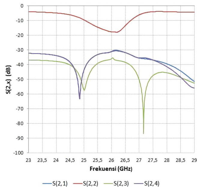
Gambar 13. Hasil S-Parameters antenna mikrostrip MIMO 4 \times 4 dengan double U-slot patch dan DGS elemen ke-2.
