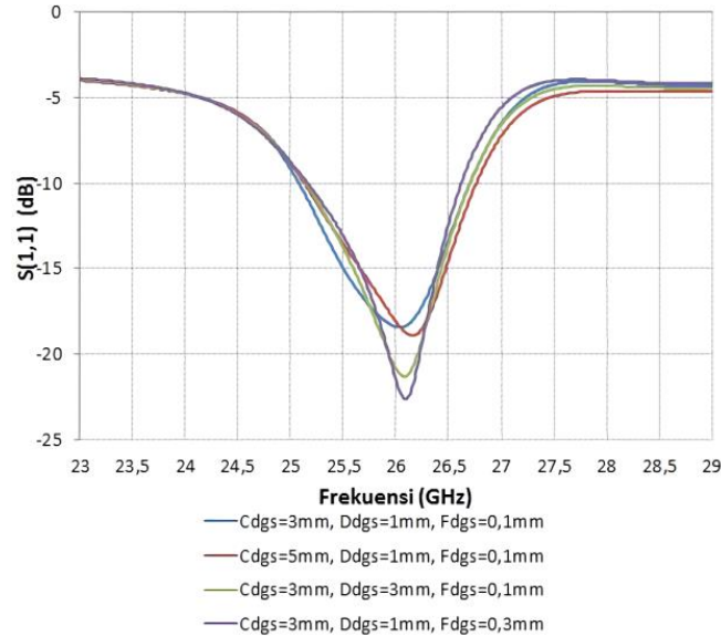
Gambar 8. Optimasi S (1,1) antenna mikrostrip tunggal dengan double U-slot patch dan DGS.
