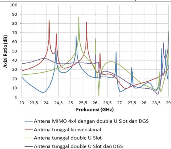
Gambar 17. Grafik axial ratio antenna mikrostrip tunggal dan MIMO 4×4.
