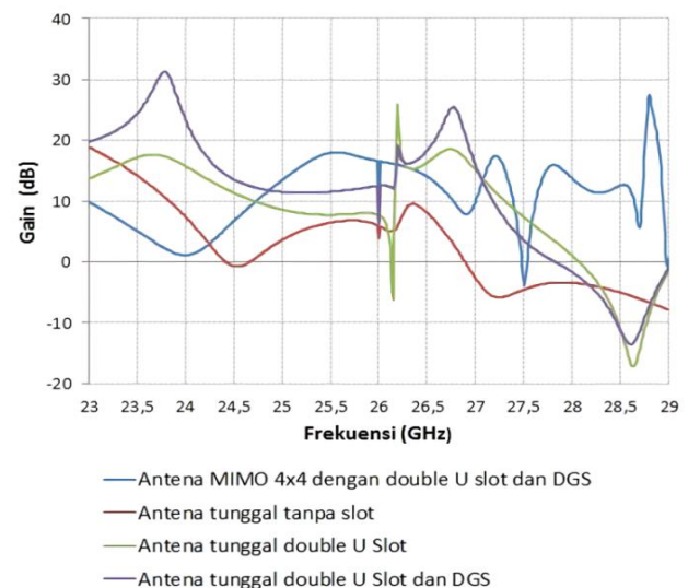
Gambar 18. Grafik gain antenna mikrostrip tunggal dan MIMO 4×4.
