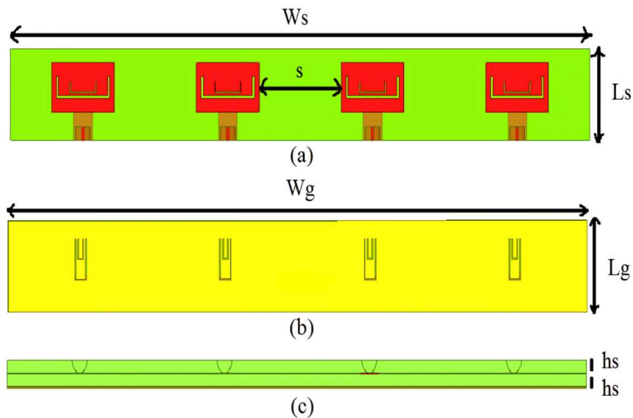
Gambar 11. (a) Bentuk antenna mikrostrip MIMO 4×4 dengan double U-slot patch dan DGS tampak atas, (b) Bentuk antenna mikrostrip MIMO 4×4 dengan double U-slot patch dan DGS tampak bawah, dan (c) Bentuk antenna mikrostrip MIMO 4×4 dengan double U-slot patch dan DGS tampak samping.
