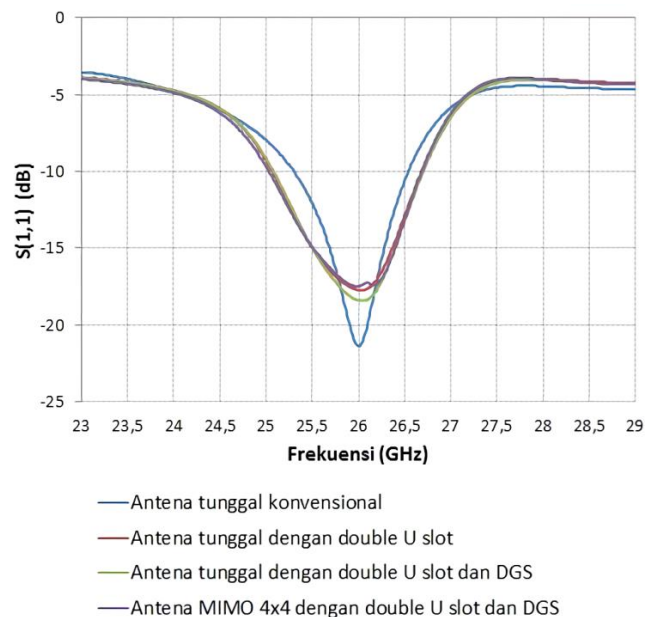
Gambar 16. Hasil S11-Parameters antenna mikrostrip tunggal dan MIMO 4×4.
