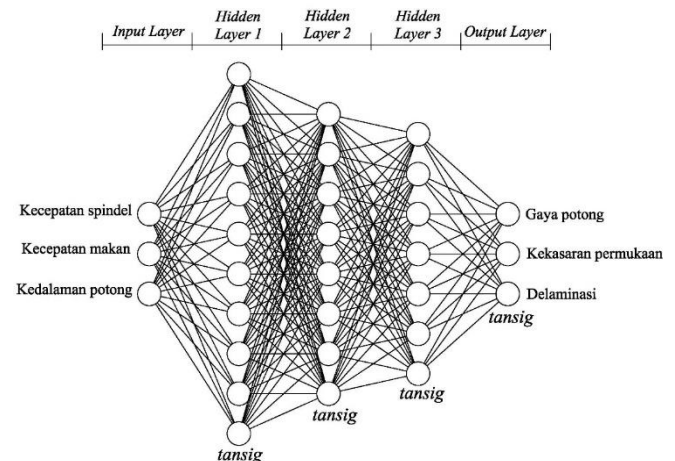
Gambar 4. Arsitektur BPNN 3-10-8-7-3.
