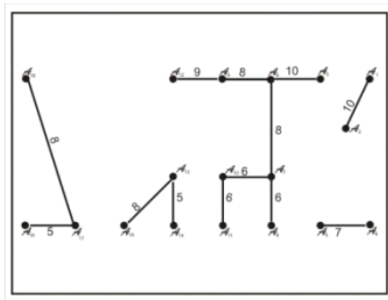
Gambar 4. Hutan F langkah 2 algoritma boruvka
