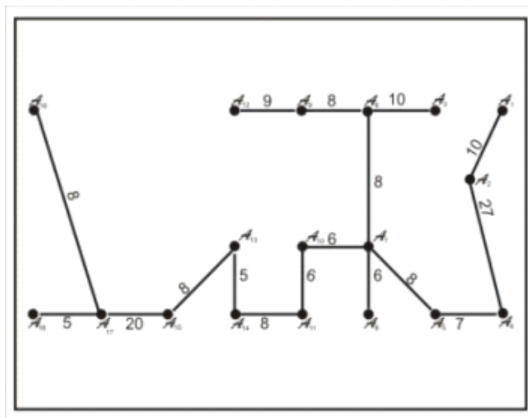
Gambar 8. Pohon perentang minmum Algoritma Solin
