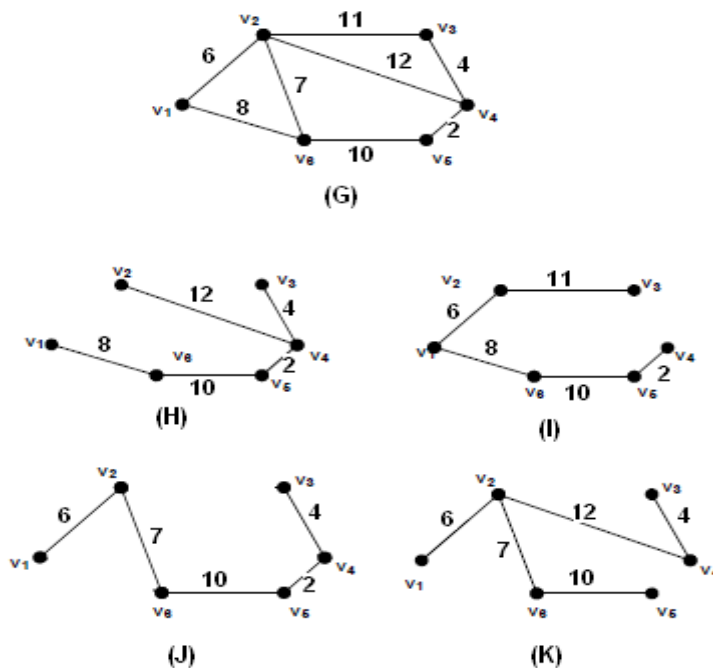
Gambar 2. Hutan. (G) graf berbobot, (H,I,J,K) pohon perentang, (J) pohon perentang minimum
