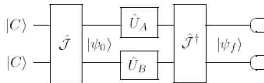
Gambar 1 Skema EWL untuk dua pemain [6]
