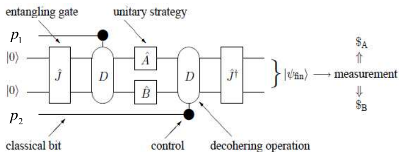
Gambar 2 Kuantum permainan untuk dua pemain dengan menggunakan skema EWL dengan mempertimbangkan faktor dekoherensi [19]
