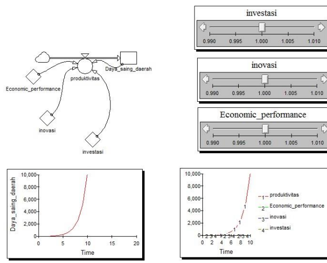
Gambar 2. Simulasi Flow Rate Konstanta Stabil
