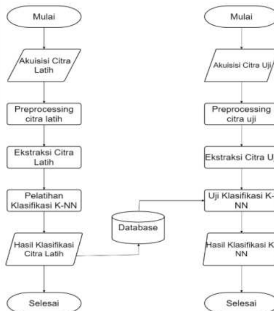
Gambar 2. Klasifikasi K-NN
