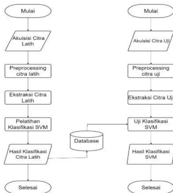
Gambar 3. Klasifikasi SVM
