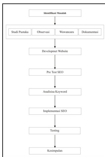
Gambar 2. Langkah Penelitian
