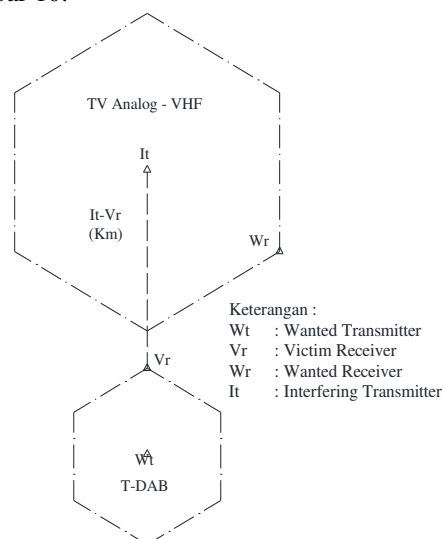
Gambar 10. Skenario TV analog menginterferensi T-DAB
