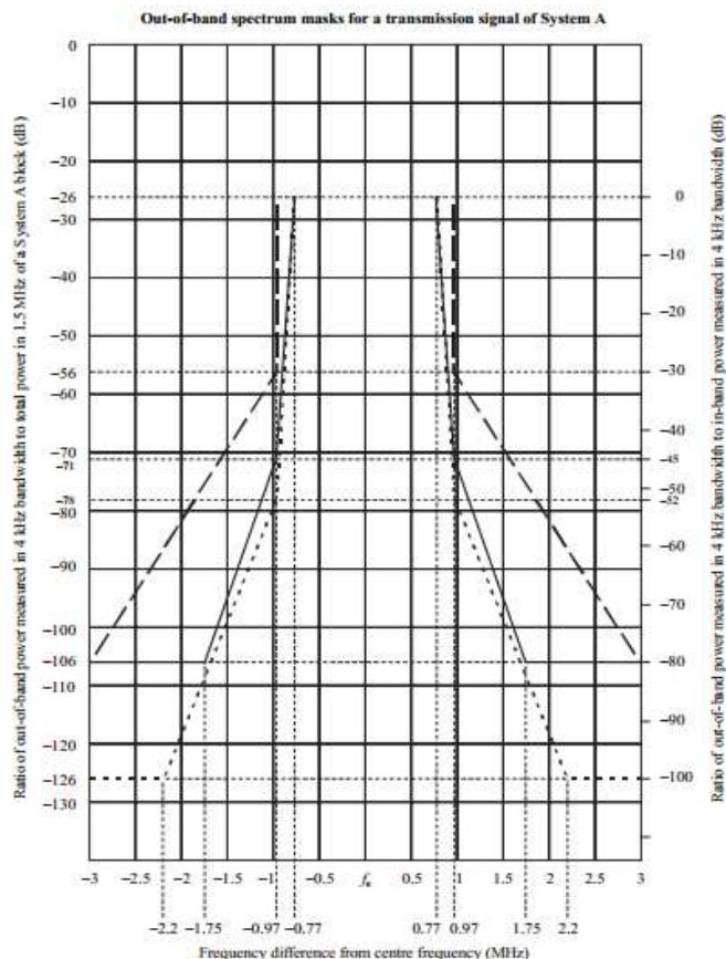
Gambar 8. Out-of-band spectrum mask T-DAB pada pita VHF(ITU-R BS.1660-6, 2012)
