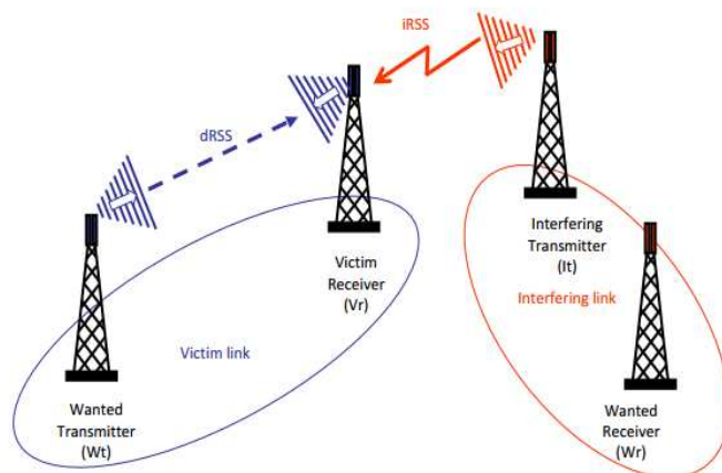
Gambar 7. Skenario victim dan interferer untuk percobaan simulasi Monte Carlo (ECO, 2010)
