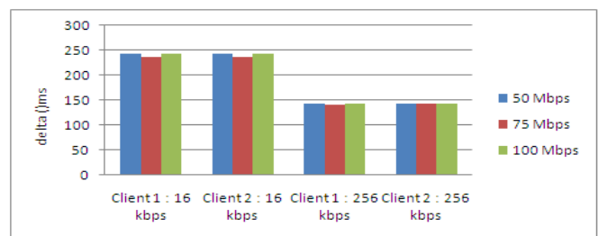
Gambar 5. Grafik Nilai Delta Skenario 3
