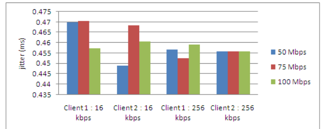
Gambar 8. Grafik Nilai Jitter Skenario 3
