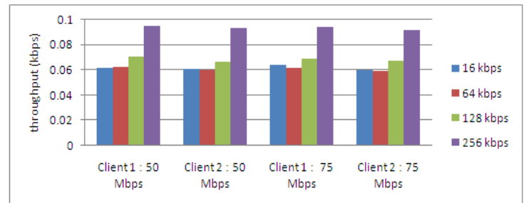
Gambar 13. Grafik Throughput Skenario 2
