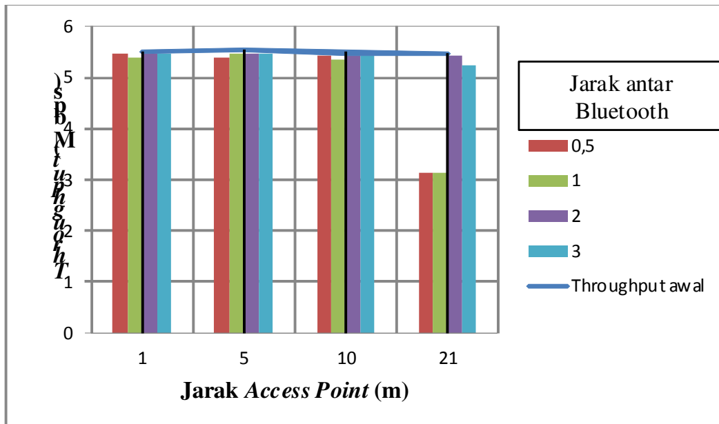
Gambar 10. Grafik Perbandingan Throughput awal Wi-Fi dengan saat ada Bluetooth
