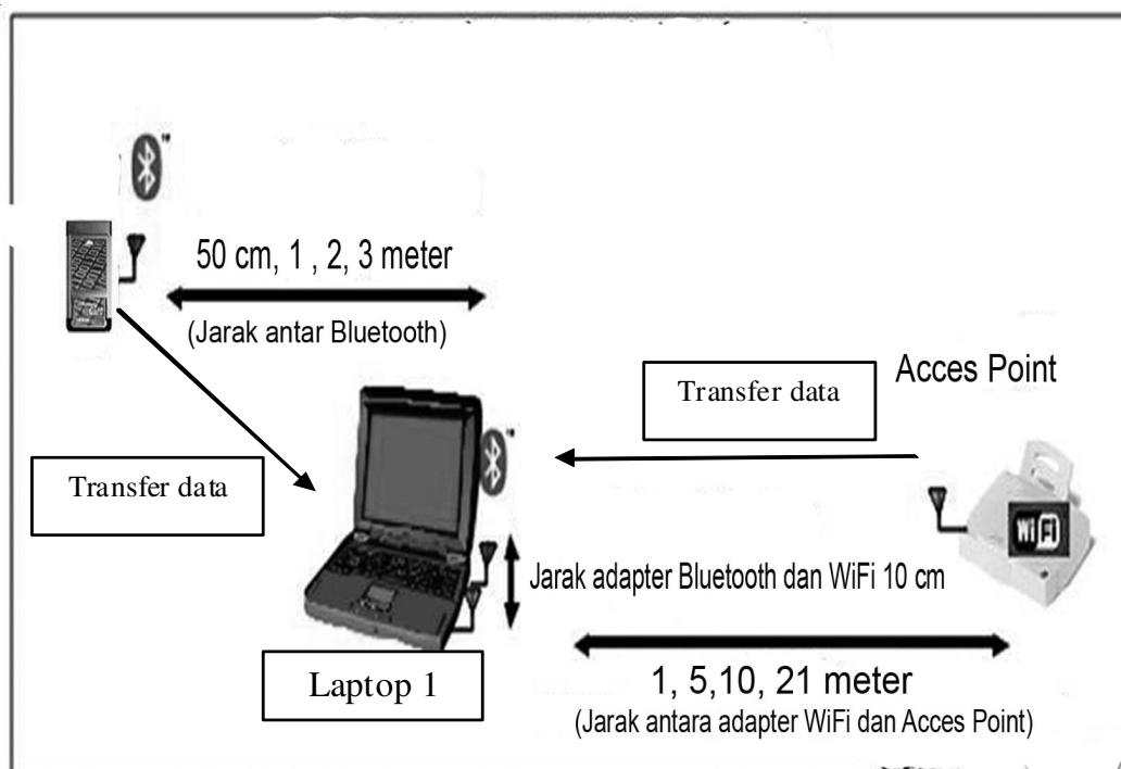
Gambar 7. Skenario Pengukuran Throughput Bluetooth dan WiFi
