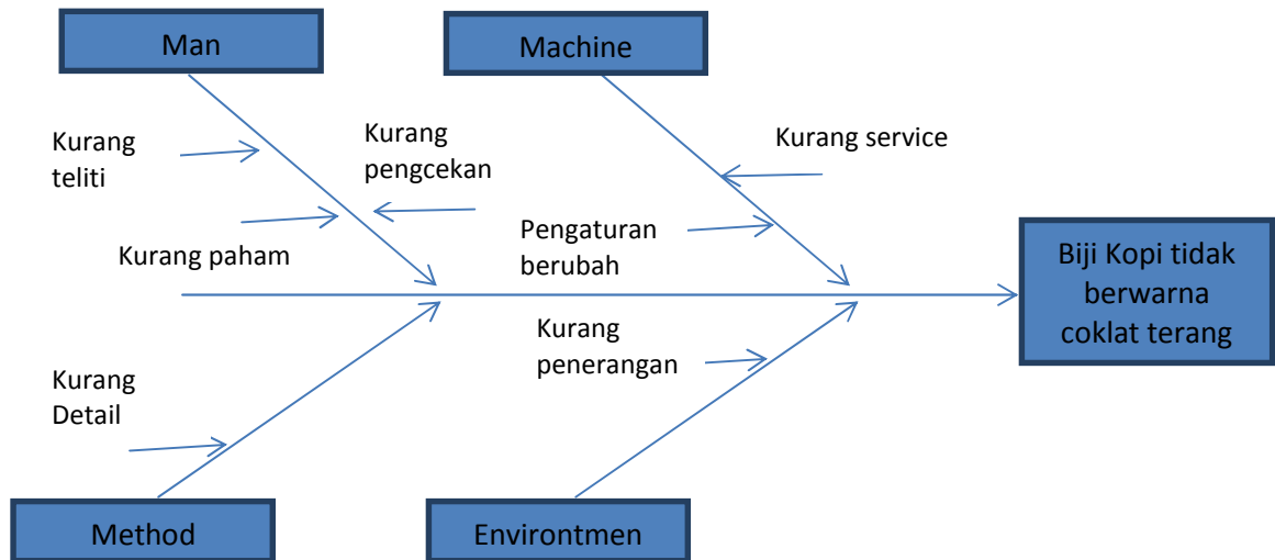
Gambar 2. Fishbone Diagram Produk Cacat Biji Kopi Tidak Berwarna Coklat Terang
