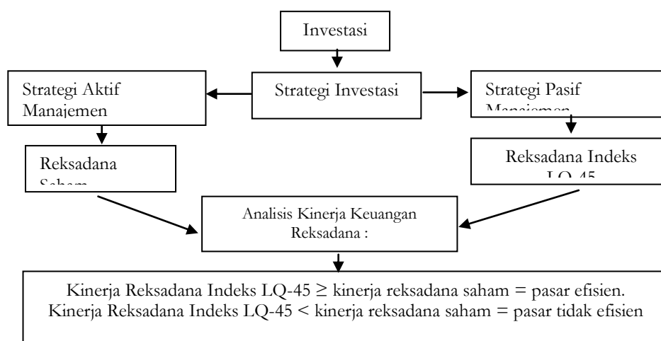
Gambar 1. Kerangka pikir
