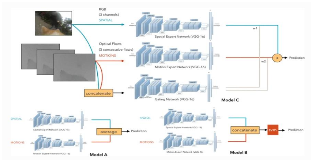
Gambar 9. Model Deep Learning dalam mendeteksi aksi manusia dalam video [20]
