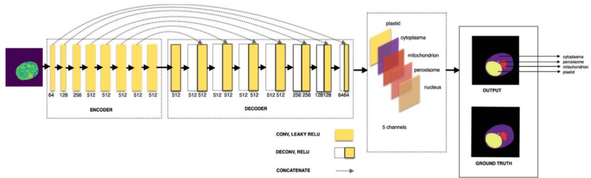
Gambar 10. Model Deep Learning dalam melakukan segmentasi sel (Sumber: [22])
