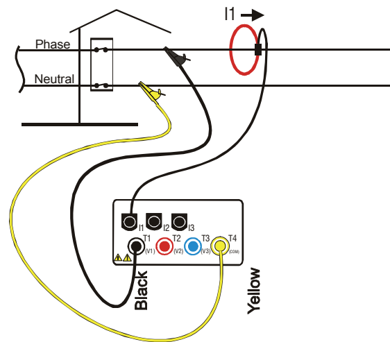
Gambar 10. Rangkaian Pengukuran Satu Phasa
