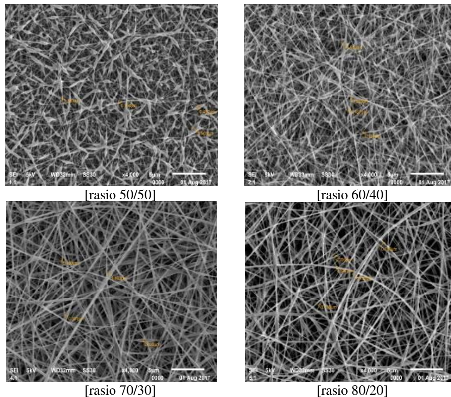
Gambar 5. Citra SEM ukuran serat hasil electrospinning PVA/gelatin (Pembesaran 4000 kali)
