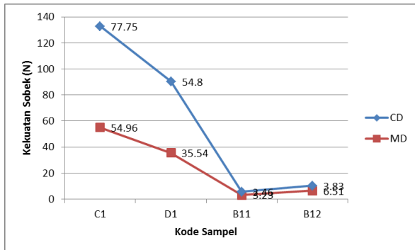
Gambar 8. Grafik kekuatan sobek geotekstil gramasi 300 g/m 2
