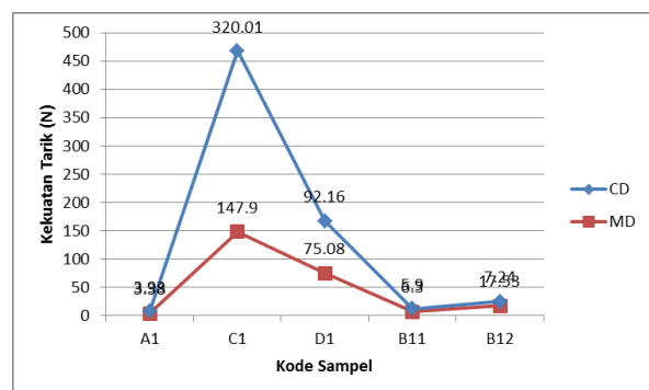
Gambar 5. Grafik kekuatan tarik geotekstil gramasi 300 g/m 2
