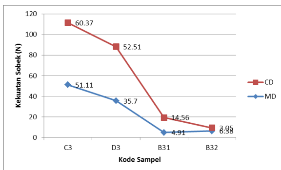
Gambar 10. Grafik kekuatan sobek geotekstil gramasi 500 g/m 2
