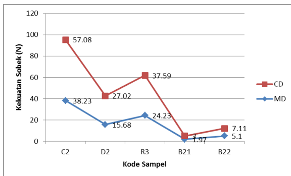
Gambar 9. Grafik kekuatan sobek geotekstil gramasi 400 g/m 2
