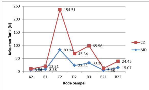
Gambar 6. Grafik kekuatan tarik geotekstil gramasi 400 g/m 2
