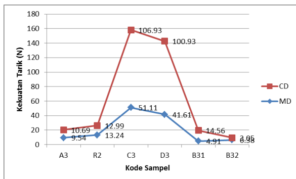
Gambar 7. Grafik Kekuatan Tarik Geotekstil Gramasi 500 g/m 2
