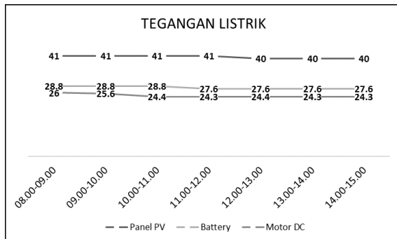
Gambar 8. Tegangan Listrik Dengan Beban.
