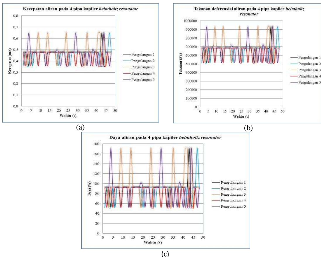
Gambar 9. Grafik percobaan 4 pipa kapiler (a) kecepatan aliran, (b) tekanan diferensial aliran, (c) daya aliran
