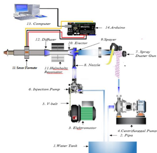
Gambar 4. Rancangan Penelitian
