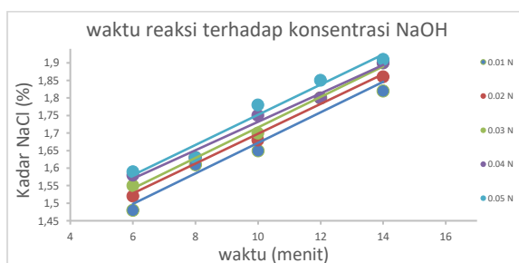
Gambar 3. Pengaruh Waktu Reaksi Terhadap Kadar Natrium Klorida (NaCl) pada Pelbagai Konsentrasi Natrium Hidroksida (NaOH)
