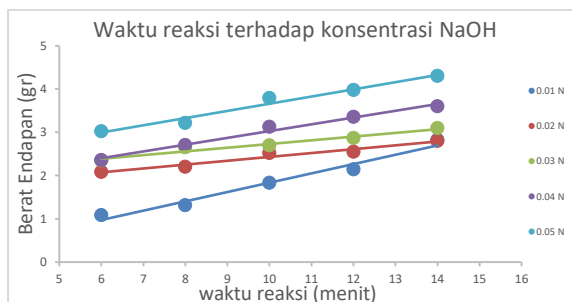
Gambar 5. Hubungan Berat Endapan dengan Waktu Reaksi pada Pelbagai Konsentrasi NaOH.
