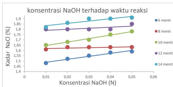
Gambar 2. Pengaruh Konsentrasi Natrium Hidroksida (NaOH) Terhadap Kadar Natrium Klorida (NaCl) pada Pelbagai Waktu Reaksi
