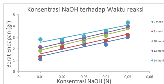
Gambar 4. Pengaruh Konsentrasi Natrium Hidroksida (NaOH) Terhadap Berat Endapan pada Pelbagai Waktu Reaksi.
