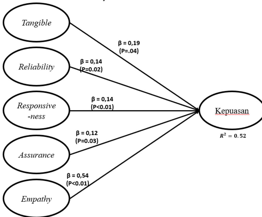
Gambar 2. Analisis Koefisien Jalur
