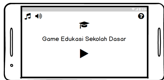
Gambar 3 Halaman Utama
