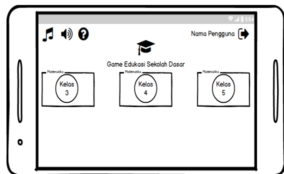
Gambar 4 Menu Utama
