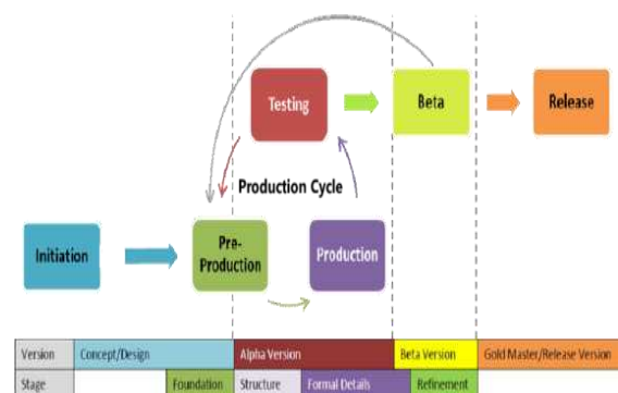
Gambar 1 Tahapan GDLC
