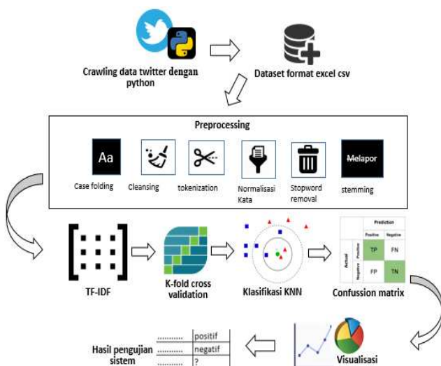
Gambar. 1. Desain sistem analisis sentimen terhadap peresepakbolaan Indonesia
