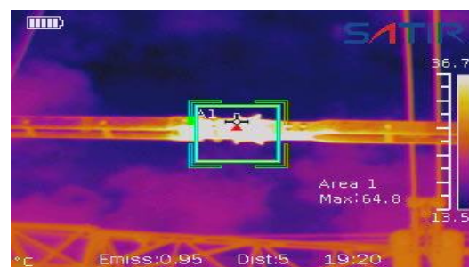
Gambar 4. hasil thermovisi sebelum perbaikan fasa T
