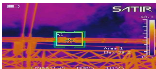
Gambar 6. hasil thermovisi setelah perbaikan Fasa R
