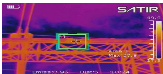
Gambar 7. hasil thermovisi setelah perbaikan Fasa S
