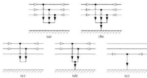
Gambar 6. Gangguan Hubung Singkat (a) HS. 3 Fasa, (b) HS. 3 Fasa-N, (c) HS. 2 Fasa, (d) HS. 2 Fasa-N, (e) HS. 1 Fasa-N.
