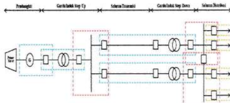
Gambar 1. Zona Proteksi.
