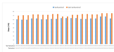
Gambar 14. Grafik pengukuran arus difasa S
