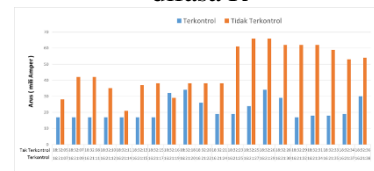
Gambar 11. Grafik pengukuran arus difasa R
