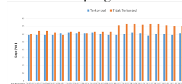
Gambar 12. Grafik pengukuran daya difasa R
