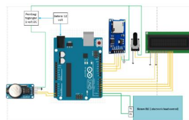
Gambar 7. Skema rangkaian data logger
