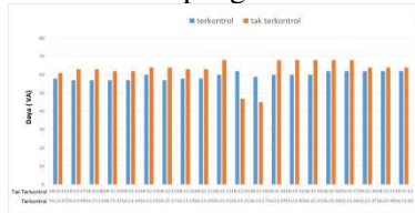
Gambar 15. Grafik pengukuran daya difasa S
