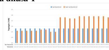
Gambar 16. Grafik pengukuran tegangan difasa T
