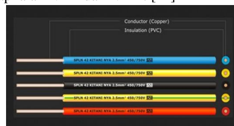
Gambar 2.8. Kabel NYA
