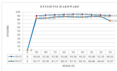
Gambar 3.1 Kurva efisiensi Hardware
