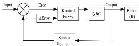
Gambar 2.1 Diagram Blok Rangkaian
