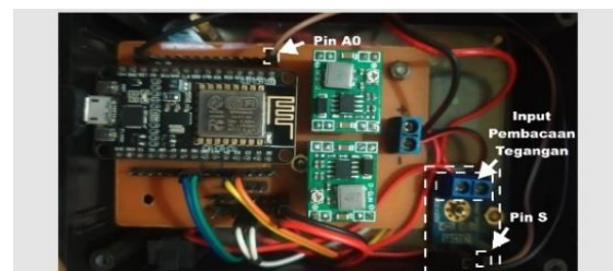
Gambar 9. Rangkaian modul voltage sensor pada kursi roda elektrik
