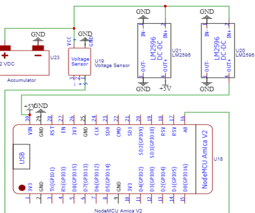
Gambar 12. Skema rangkaian sensor tegangan
