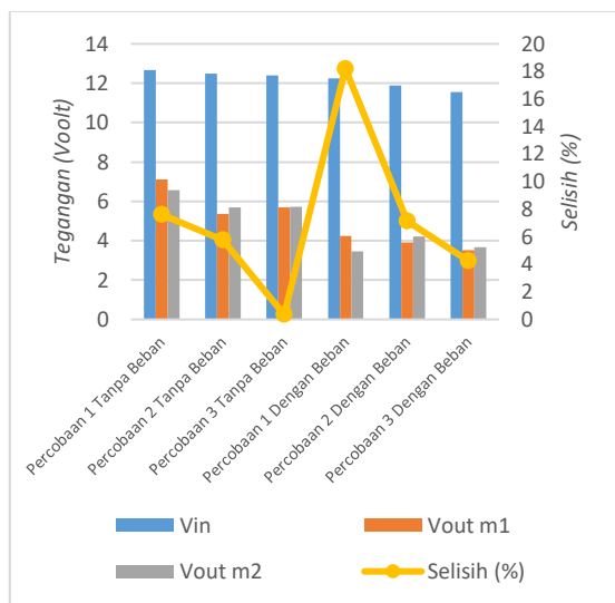
Gambar 15. Grafik tegangan catu daya motor DC
