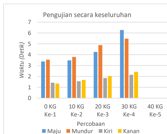
Gambar 21. Grafik pengujian secara keseluruhan
