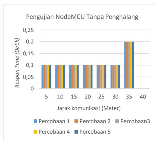
Gambar 17. Grafik pengujian NodeMCU tanpa penghalang
