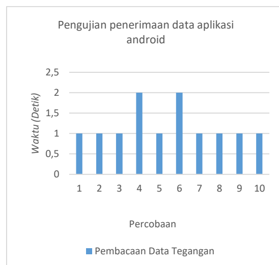
Gambar 20. Grafik penerimaan data dari aplikasi android
