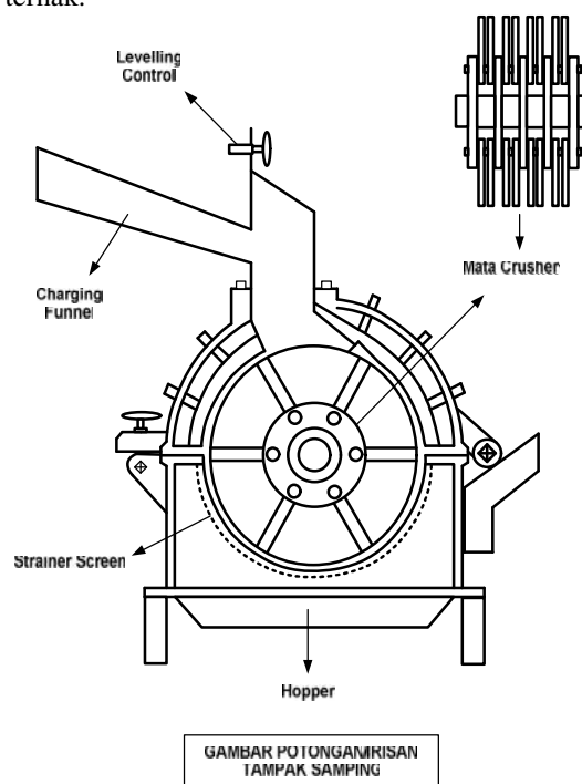
Gambar 1. Alat pengolah limbah ikan
