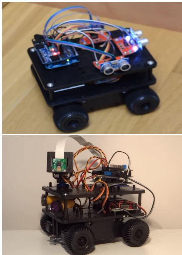
Gambar 1. Model robot yang dibangun
