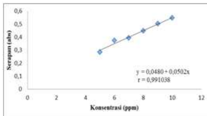
Gambar 1. Grafik Kurva Baku Kafein
