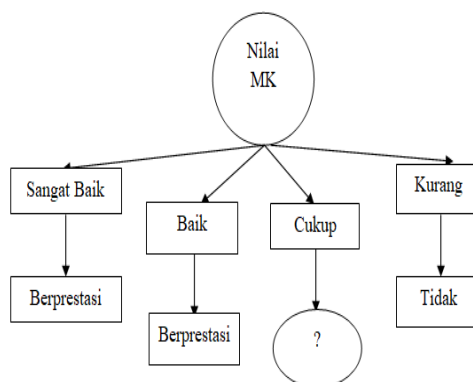
Gambar 6. Pohon Keputusan 1
