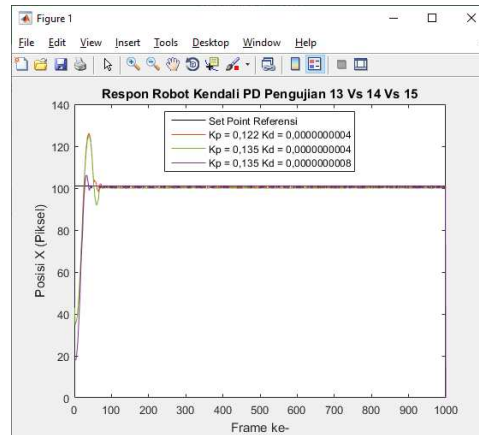
Gambar 15. Grafik Respons Robot Pengujian 13, 14 dan 15
