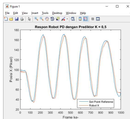
Gambar 20. Respons Robot dengan Prediktor
