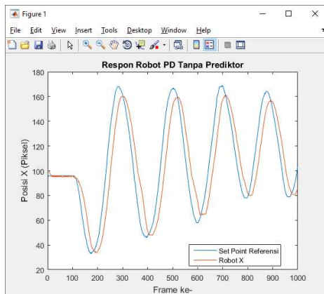
Gambar 19. Respons Robot Tanpa Prediktor
