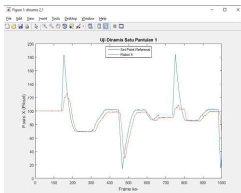
Gambar 23. Grafik Respons Uji Dinamis Kondisi 2
