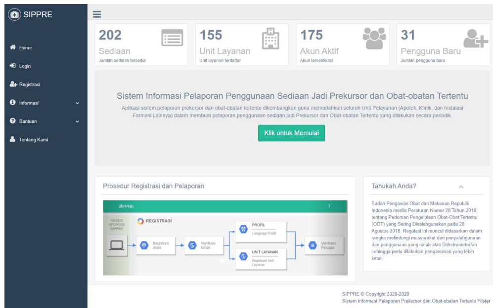
Gambar. 8. Desain Antarmuka Halaman Awal
