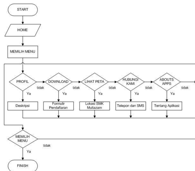
Gambar 4.1. Flowchart aplikasi SMK Multazam
