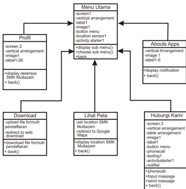
Gambar 4.3. Class Diagram aplikasi SMK Multazam
