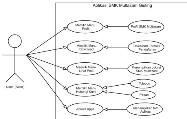
Gambar 4.2. Use Case Diagram aplikasi SMK multazam
