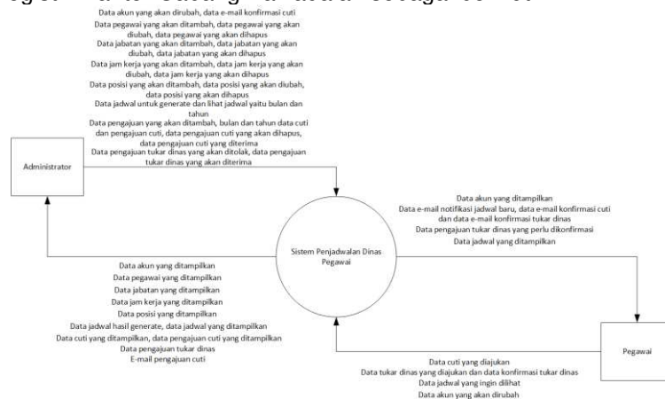
Gambar 2. Diagram Konteks
