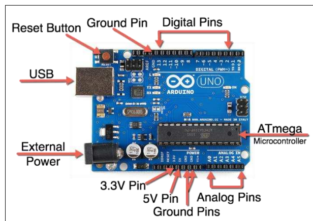
Figure 4. Arduino Uno
