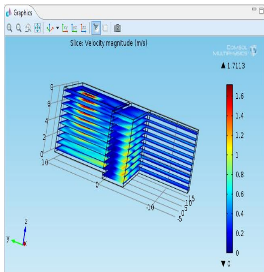
Gambar 4. Distribusi kecepatan udara dengan nilai input 1.73 m/s
