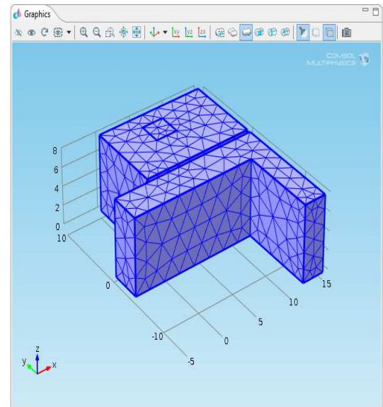
Gambar 3. Geometri yang mengalami meshing
