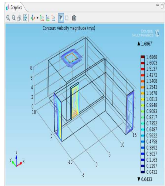
Gambar 5. Kontur kecepatan udara dengan nilai input 1.73 m/s
