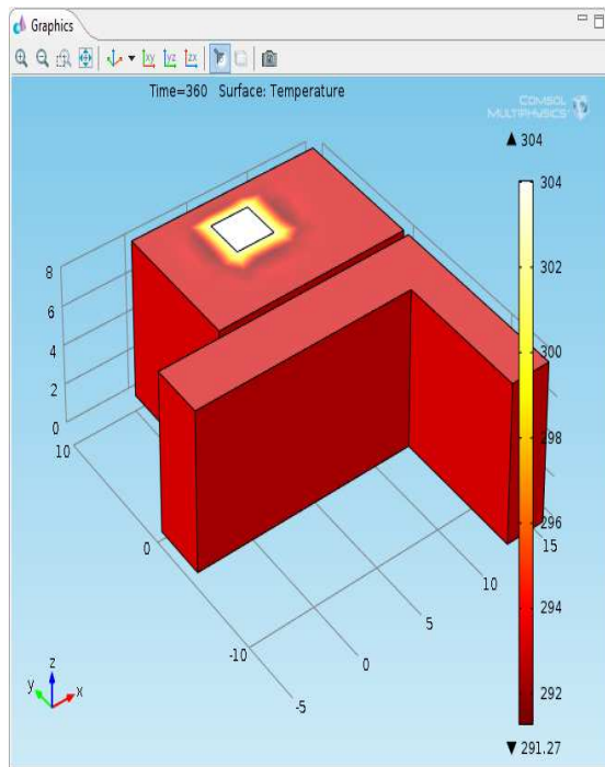
Gambar 7. Distribusi suhu udara di dalam ruangan kantor dan lorong
