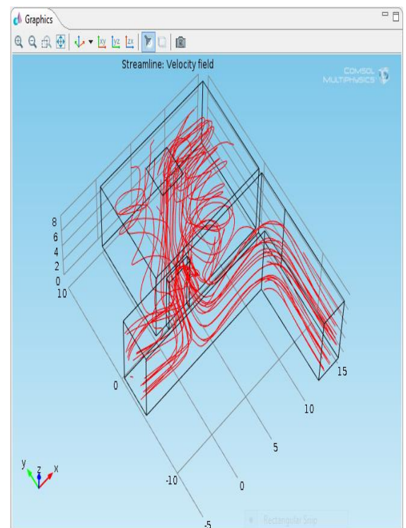
Gambar 8. Arah aliran udara pada saat kecepatan udara = 0.5 m/s
