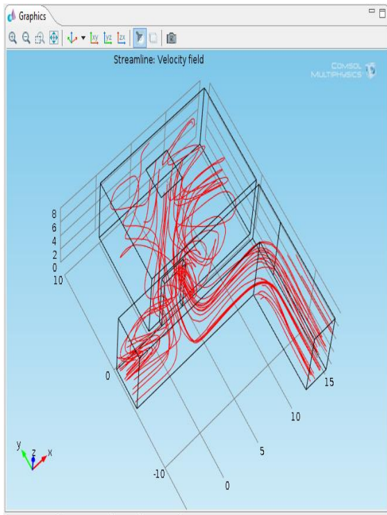
Gambar 10. Arah aliran udara pada kecepatan = 1 m/s
