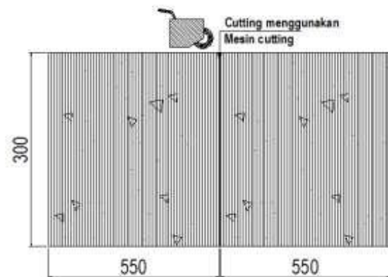
Gambar 13 Sketsa pekerjaan grooving beton
