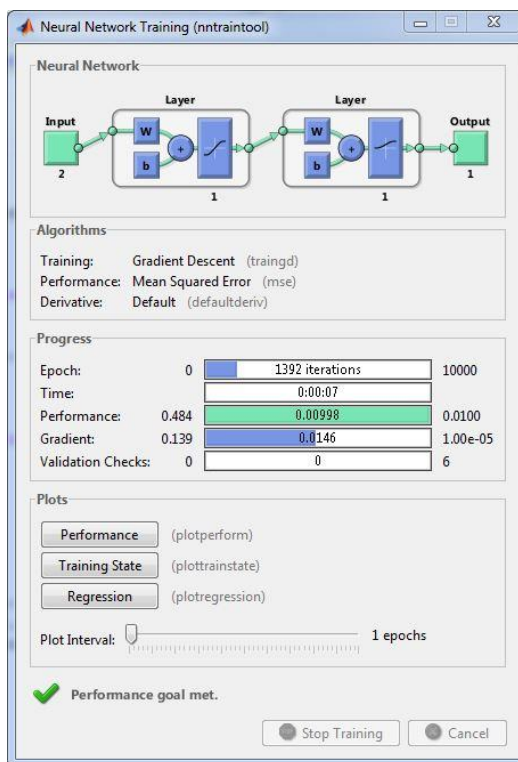
Gambar 3. Pengujian Prediksi 1 Menggunakan Arsitektur 2-1-1
