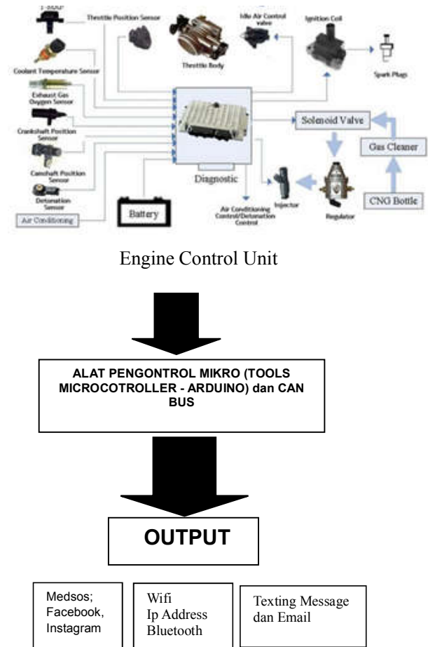
Gambar 3 Arsitektur Perancangan IoT ECU
