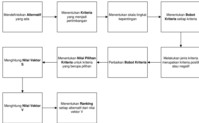
Gbr. 3. SPK dengan metode weighted product
