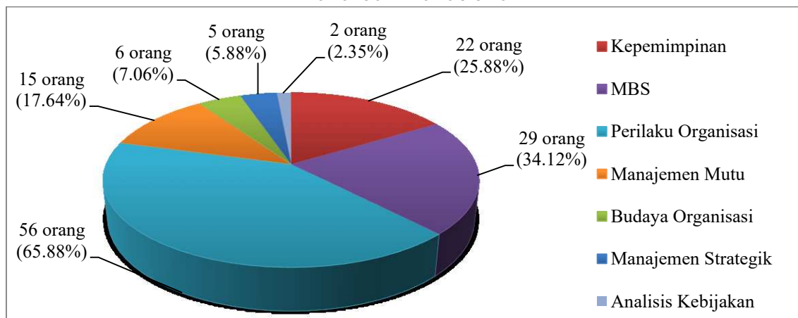
Gambar 2. Diagram Lingkaran Persentase Kecenderungan dalam Bidang Kajian Penelitian Mahasiswa
