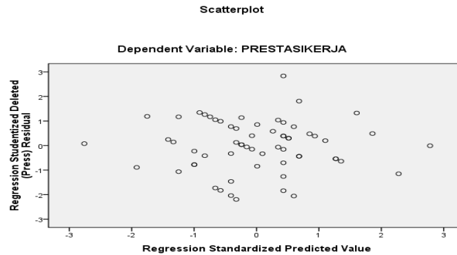
Gambar V.2. Grafik Scatterplot
