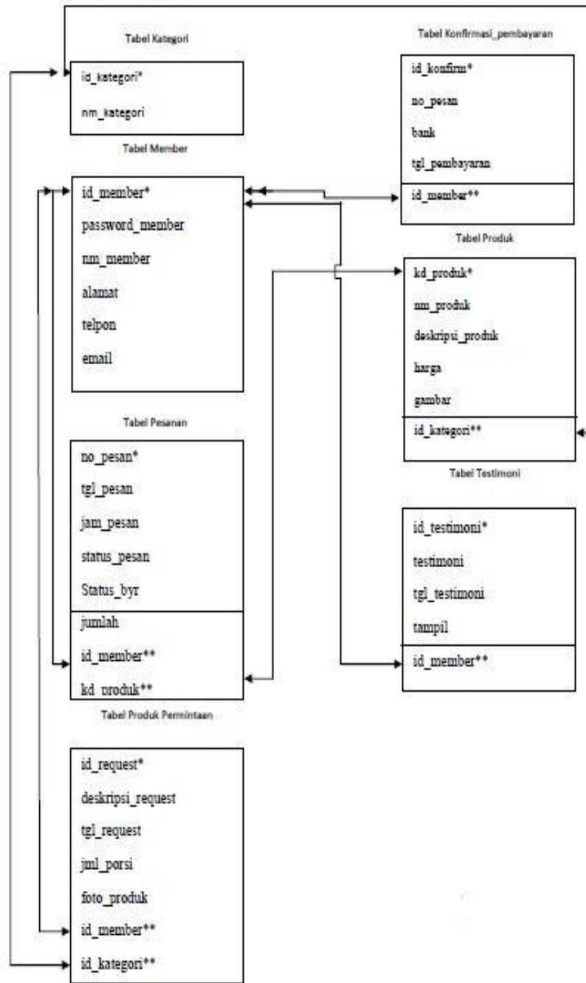
Gambar 6. Bentuk Normal Kedua
