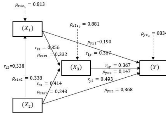
Gambar 2. Hubungan kausal variabel X_1, X_2, X_3 , dan Y
