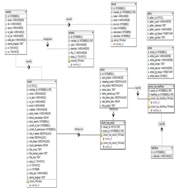
Gambar 7. Rancangan Database
