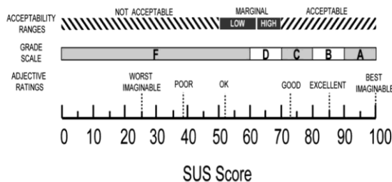
Gambar 16. Skor SUS
