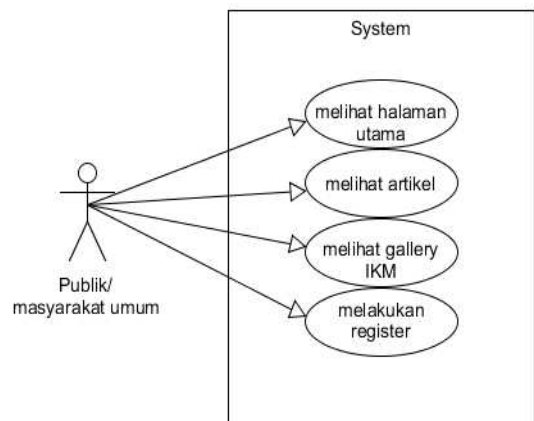
Gambar 4. Usecase Publik
